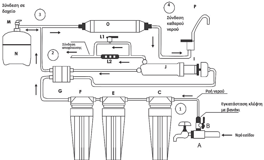
Εικόνα 1α (Αντίστροφη όσμωση 5 σταδίων)
