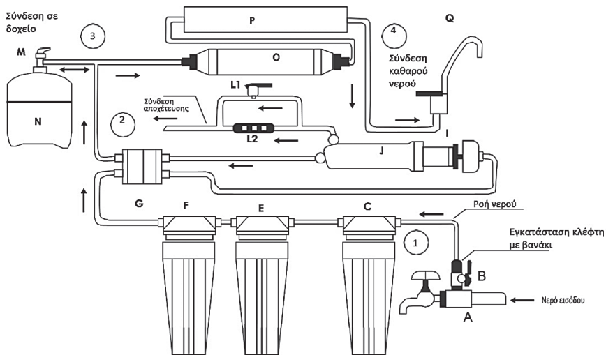
Εικόνα 1β (Αντίστροφη όσμωση 6 σταδίων)
